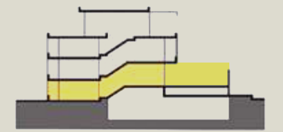
CORTE ESQUEMÁTICO
