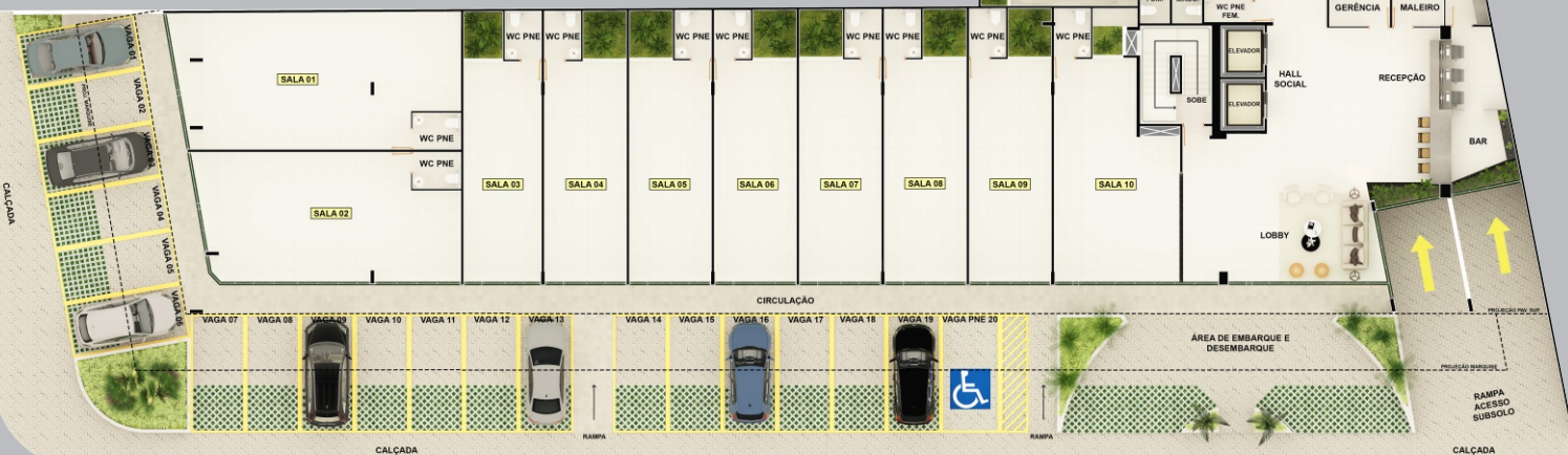
PLANTA BAIXA PAVIMENTO TÉRREO
