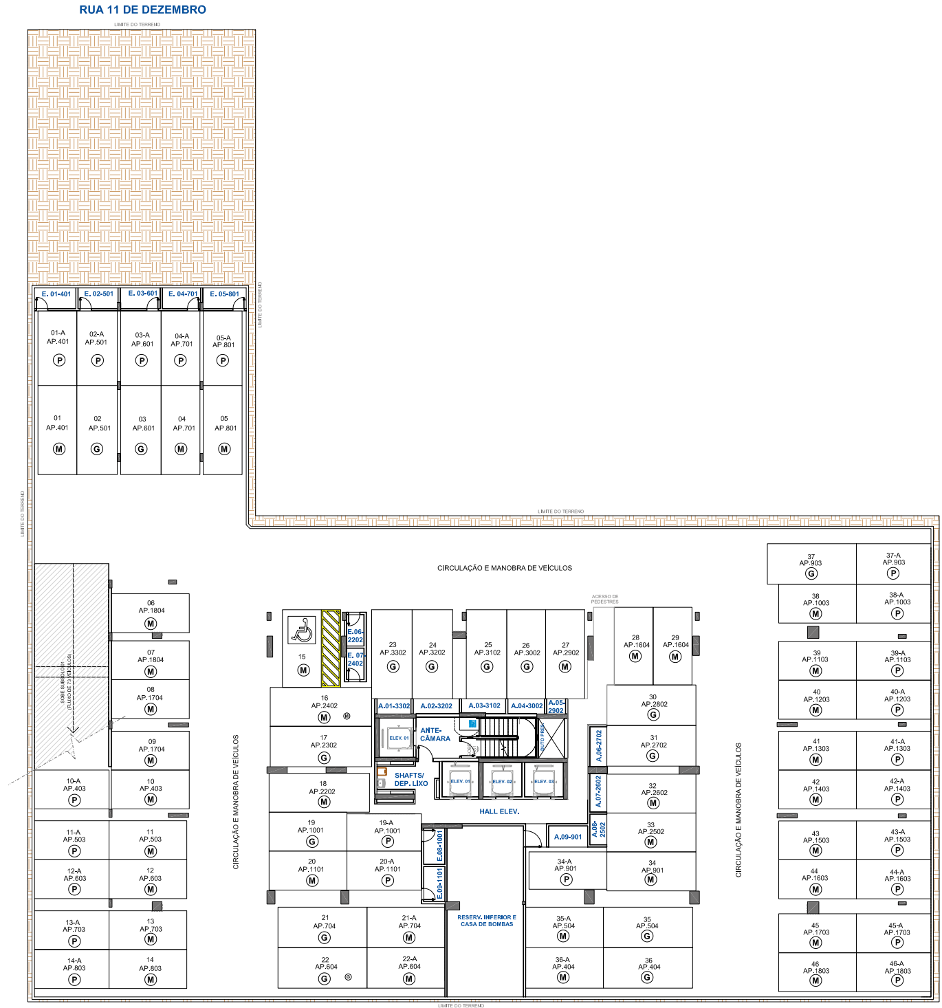
PLANTA SUBSOLO 02
