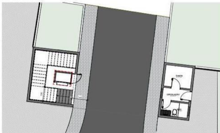
① Planta baixa - Guarita 1:50
