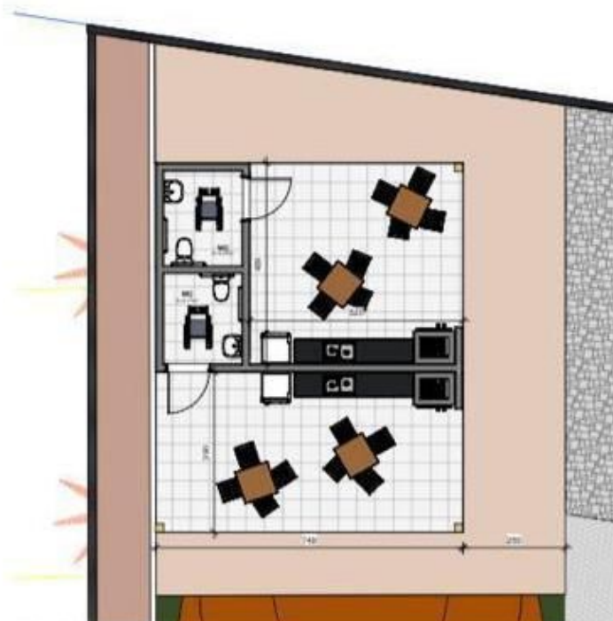
1 Planta baixa - Quiosque 1 : 50
