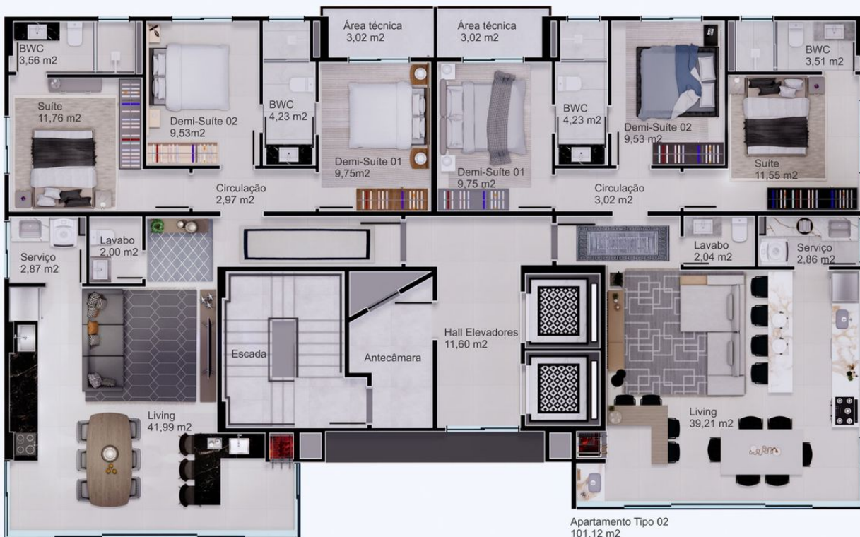
Apartamento Tipo 01 101,32 m²
