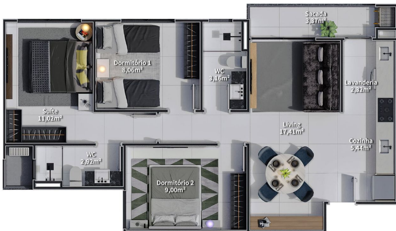
PLANTA TIPO 03 - 2º ao 15º PAVIMENTO
