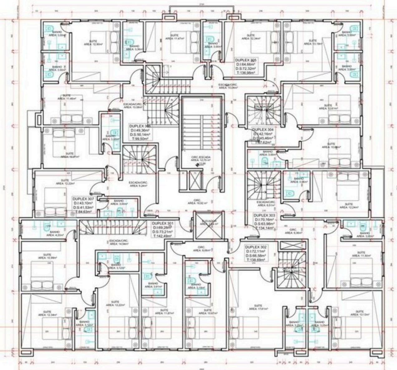
DUPLEX INFERIOR ESC. 1:75
