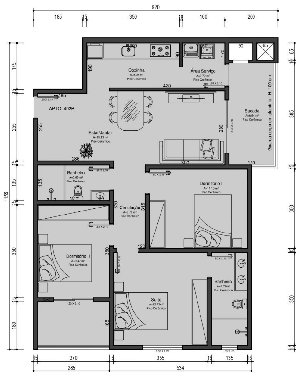
PLANTA BAIXA 4º PAVTO LAZER E TIPO DIFERENCIADO TORRE B APTO 402B
