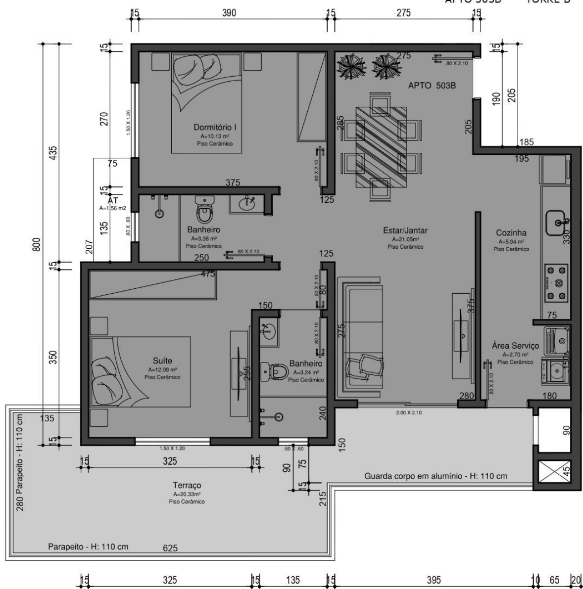
PLANTA BAIXA 5º PAVTO TIPO DIFERENCIADO TORRE B
