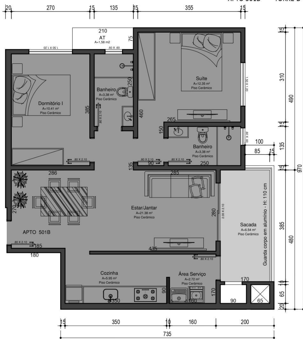
PLANTA BAIXA 5º PAVTO TIPO DIFERENCIADO TORRE B
